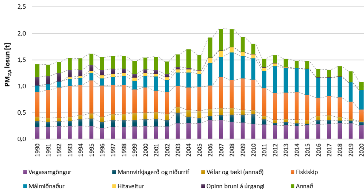
Mynd 5: Losun á svifryki (PM 2,5 ) frá 1990, skipt eftir uppsprettum losunar.
