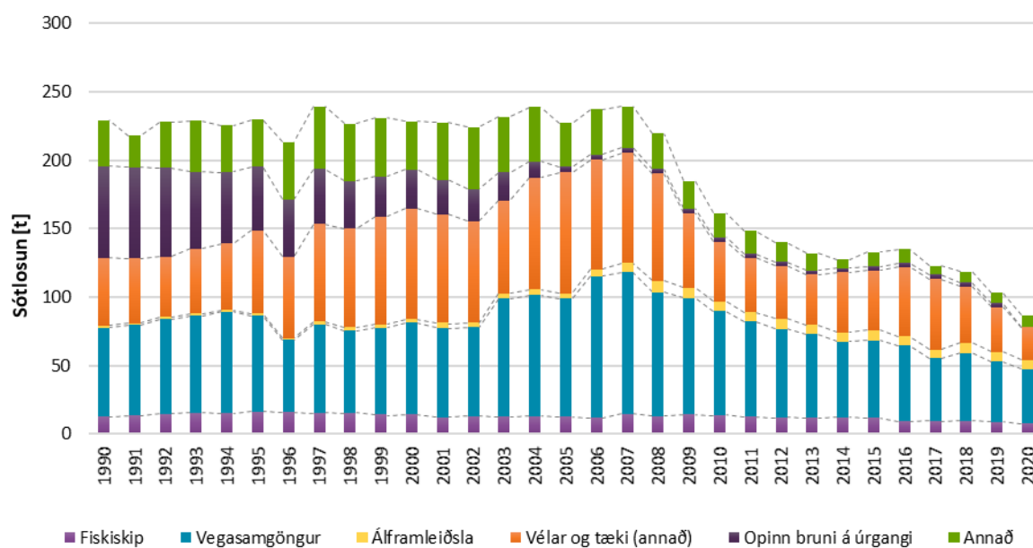
Mynd 8: Losun á sóti (BC) frá 1990, skipt eftir uppsprettum losunar
