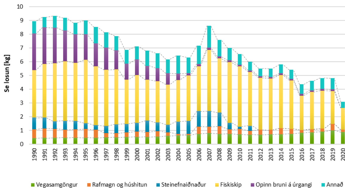
Mynd 21: Losun á selen (Se) frá 1990, skipt eftir uppsprettum losunar.
