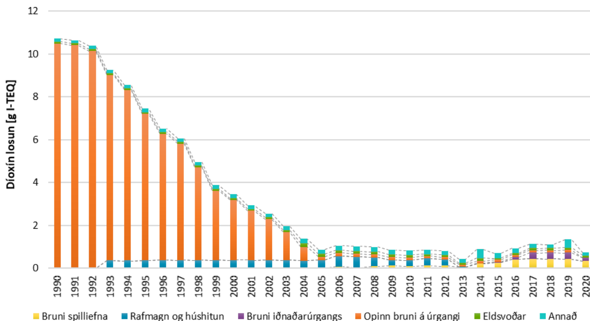
Mynd 10: Losun á díoxíni (PCDD/PCDF) frá 1990, skipt eftir uppsprettum losunar.
