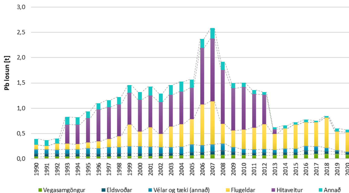
Mynd 14: Losun á blýi (Pb) frá 1990, skipt eftir uppsprettum losunar.
