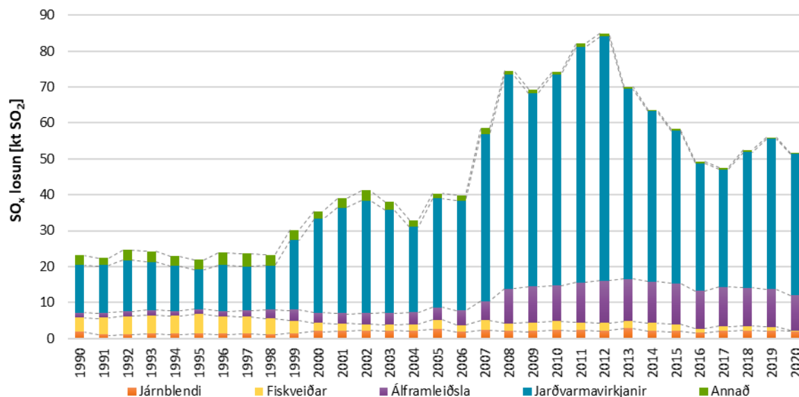
Mynd 1: Losun á brennisteinsoxíðum ( SO_x ) frá 1990, skipt eftir uppsprettum losunar. Losun H_2S frá jarðvarmavirkjunum er reiknuð yfir í SO_2 ígildi.
