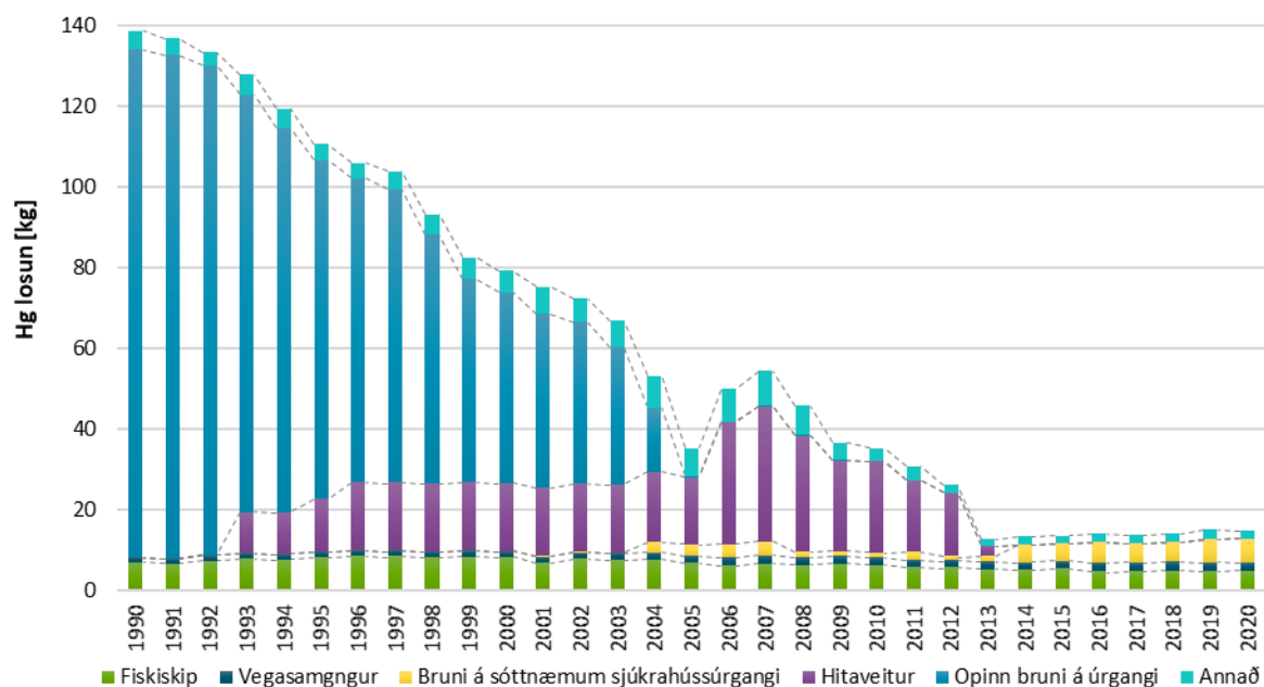
Mynd 16: Losun á kvikasilfri (Hg) frá 1990, skipt eftir uppsprettum losunar.
