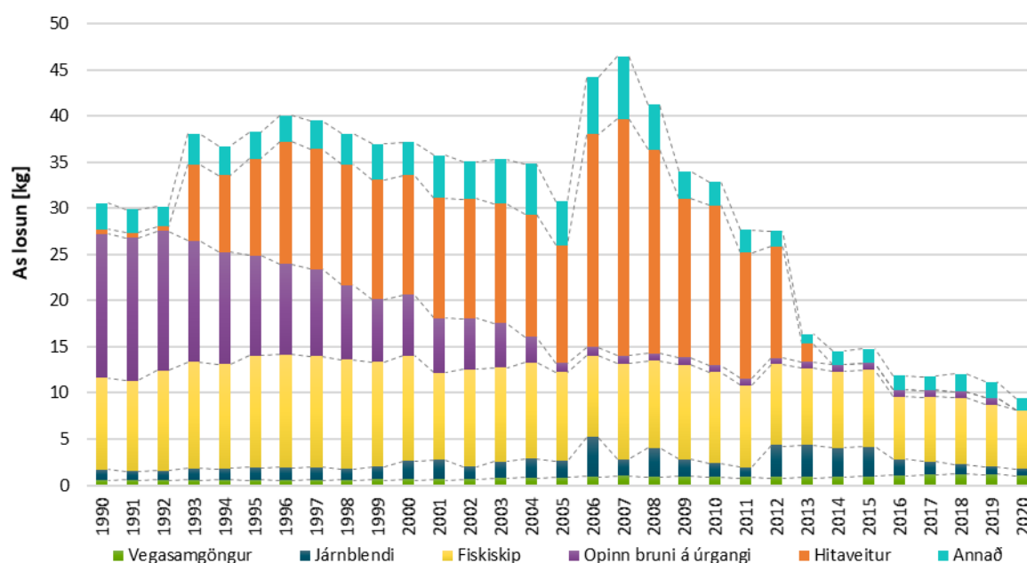
Mynd 17: Losun á arseni (As) frá 1990, skipt eftir uppsprettum losunar.
