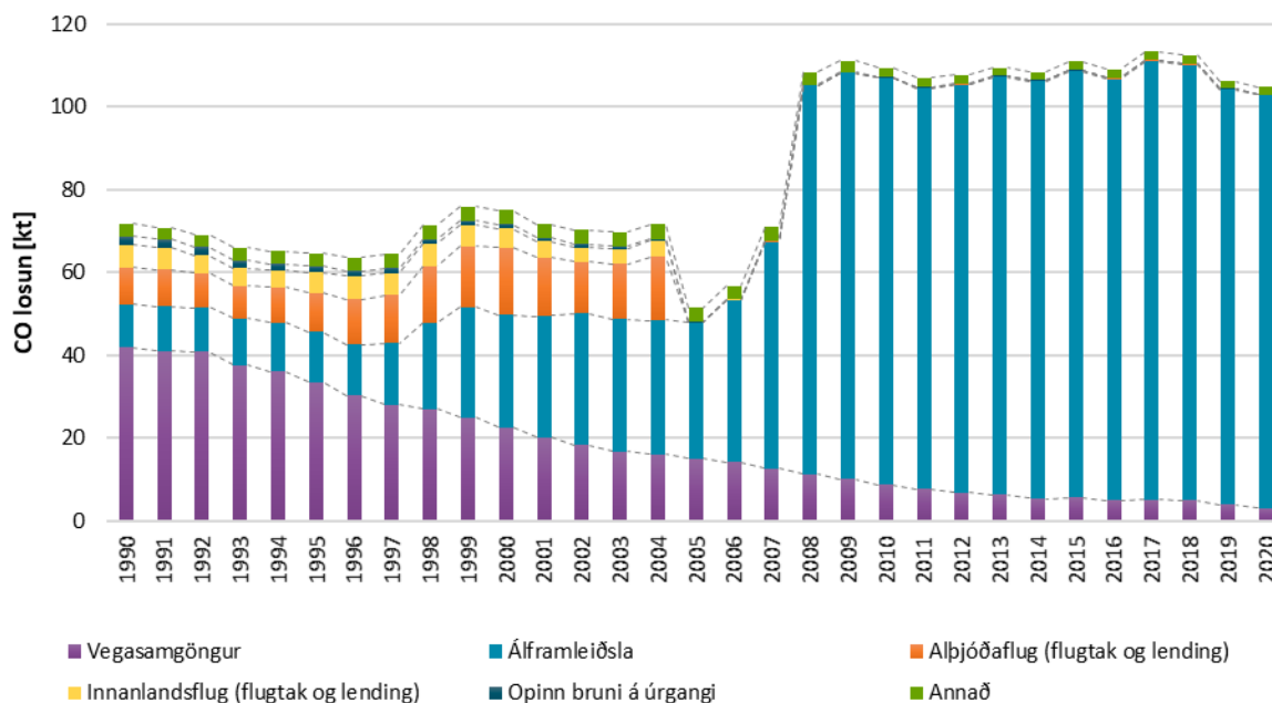
Mynd 9: Losun á kolmónoxíði (CO) frá 1990, skipt eftir uppsprettum losunar. Skyndilegur samdráttur í CO losun milli 2004 og 2005 er kominn til vegna notkunar á mismunandi gagnauppsprettum við útreikning losunar. Fyrir árin 1990-2004 er losunin metin út frá eldsneytissölum en frá 2005 er losunin metin frá gögnum frá Eurocontrol. Trúlega er ekki um raunverulega breytingu að ræða 2004-2005. Unnið er að því að betrubæta losunarreikninga fyrir flug þanngi að samræmi í tímalínunni sé til staðar.
