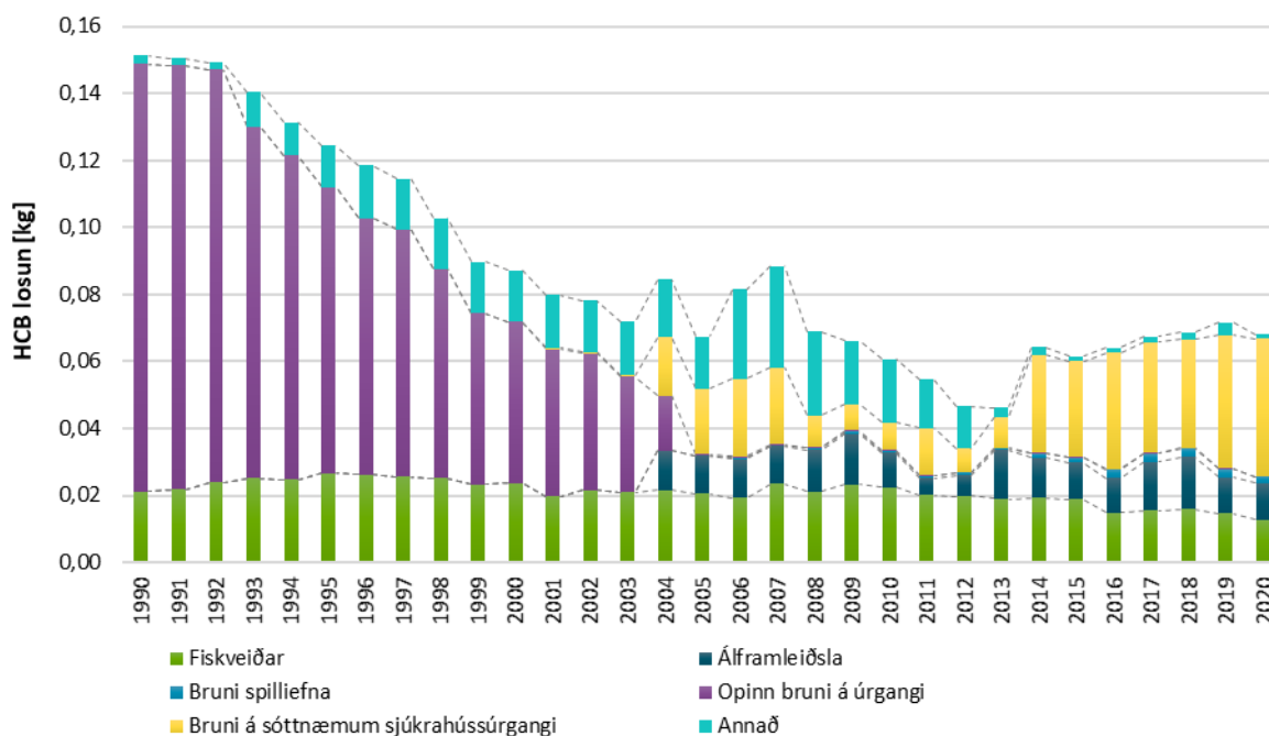
Mynd 12: Losun á hexaklórbenseni (HCB) frá 1990, skipt eftir uppsprettum losunar.
