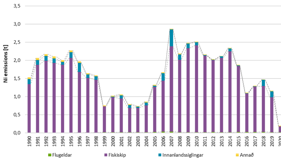
Mynd 20: Losun á nikkeli (Ni) frá 1990, skipt eftir uppsprettum losunar.
