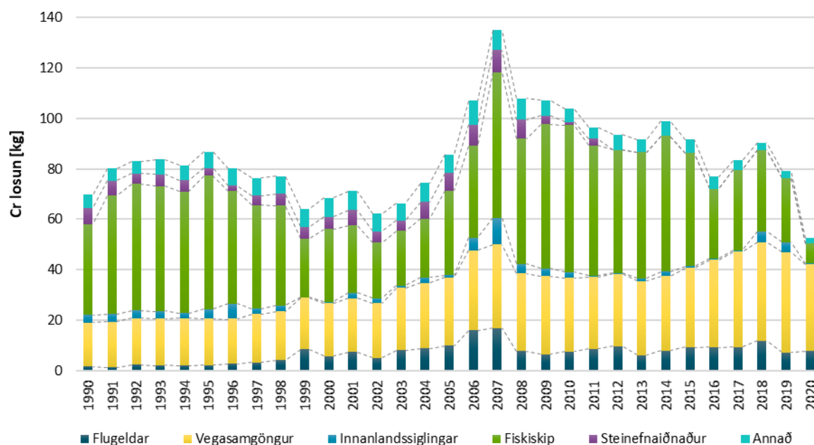
Mynd 18: Losun á krómi (Cr) frá 1990, skipt eftir uppsprettum losunar.
