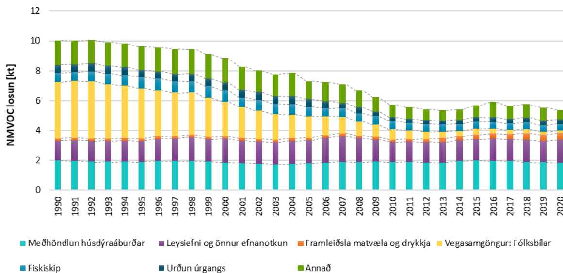
Mynd 4: Losun á rokgjörnum, lífrænum efnasamböndum (NMVOC) frá 1990, skipt eftir uppsprettum losunar.
