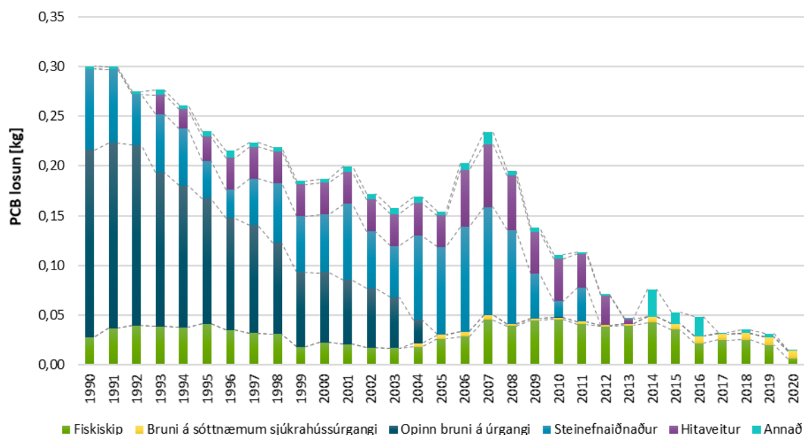
Mynd 13: Losun á póliklórbifenýlsamböndum (PCB) frá 1990, skipt eftir uppsprettum losunar.
