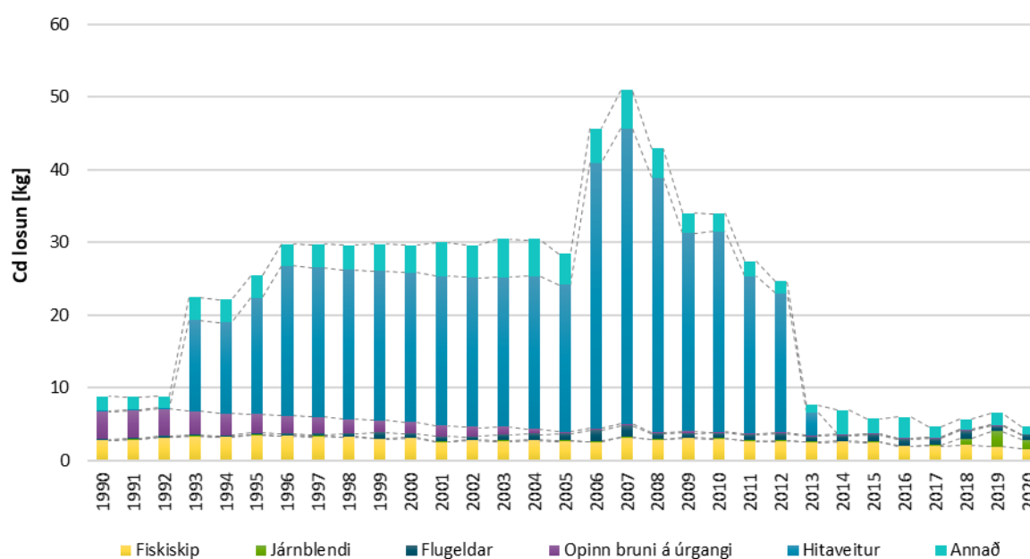
Mynd 15: Losun á kadmíni (Cd) frá 1990, skipt eftir uppsprettum losunar.
