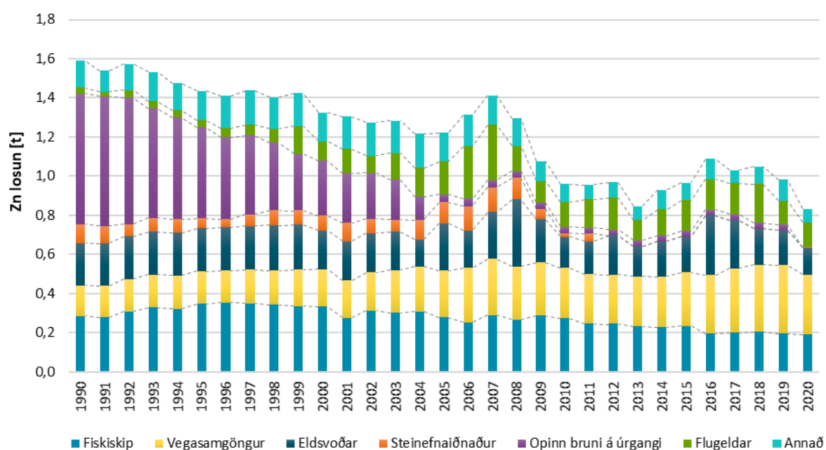
Mynd 22: Losun á sinki (Zn) frá 1990, skipt eftir uppsprettum losunar.
