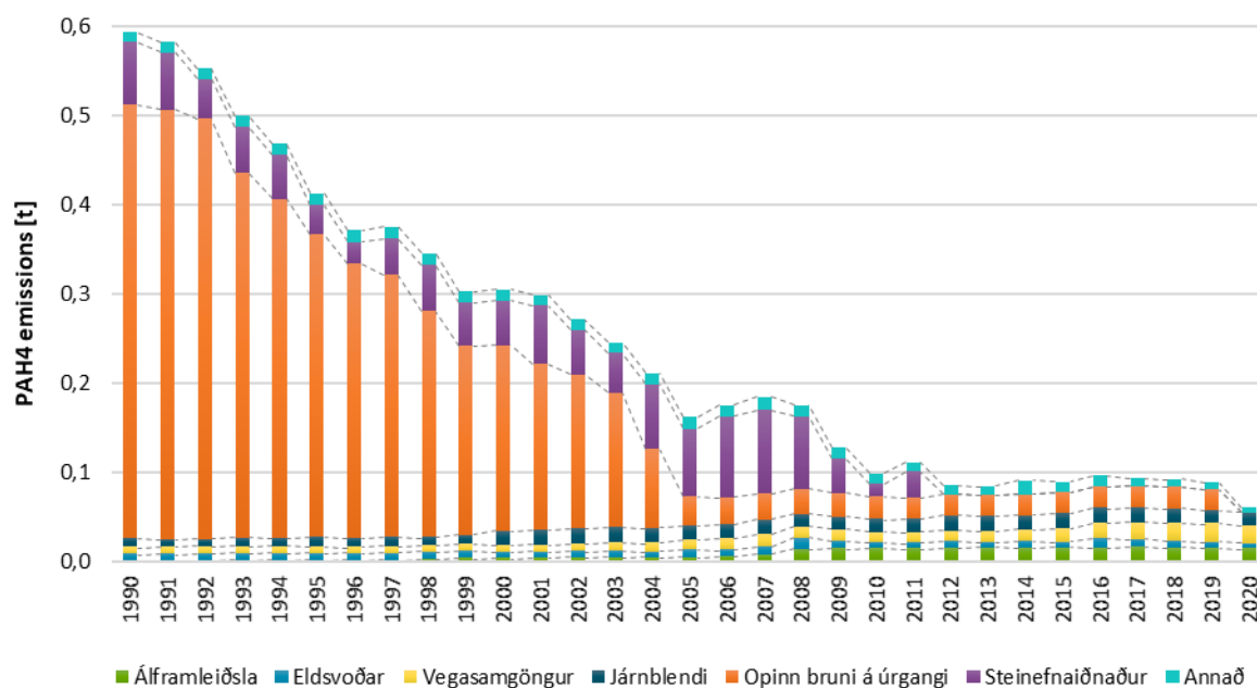
Mynd 11: Losun á fjölhringja arómatískum vetniskolefnum (PAH4) frá 1990, skipt eftir uppsprettum losunar.
