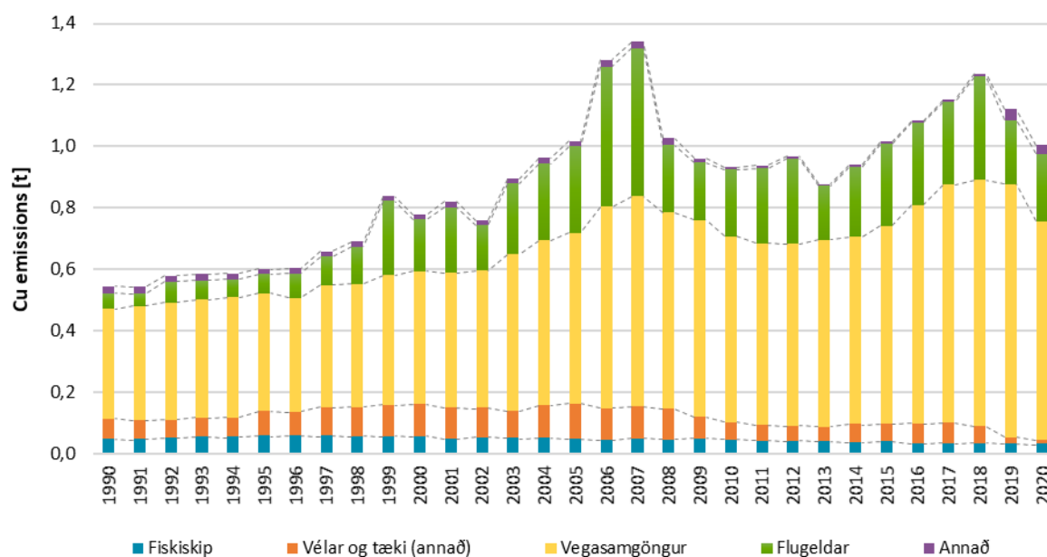
Mynd 19: Losun á kopar (Cu) frá 1990, skipt eftir uppsprettum losunar.
